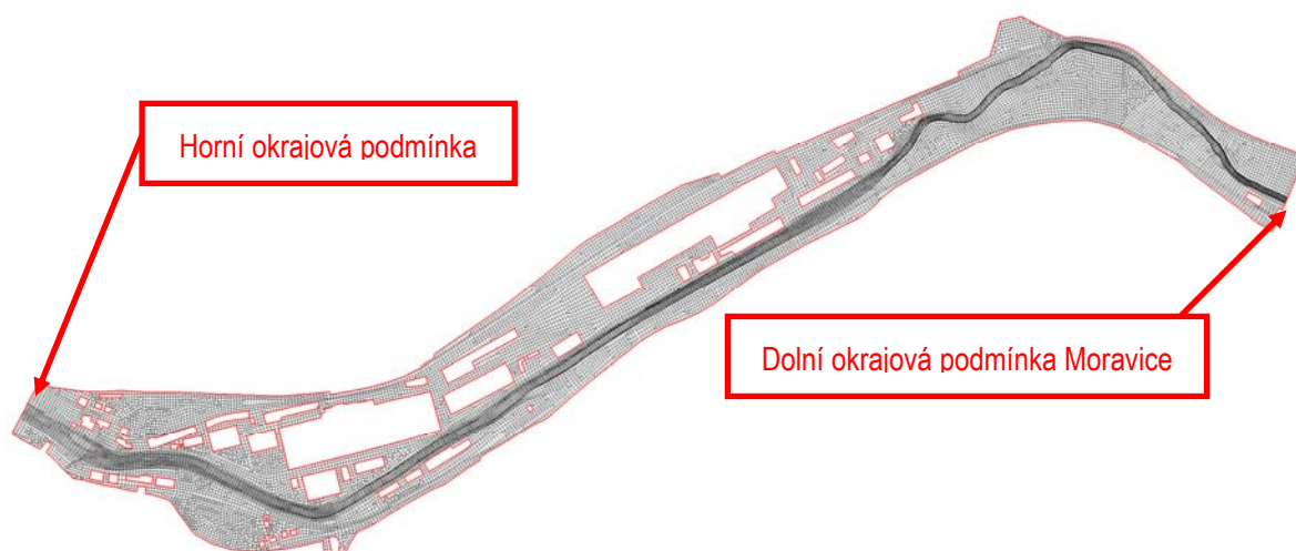
Obrázek 3 – Schéma výpočetní sítě modelu Moravice
